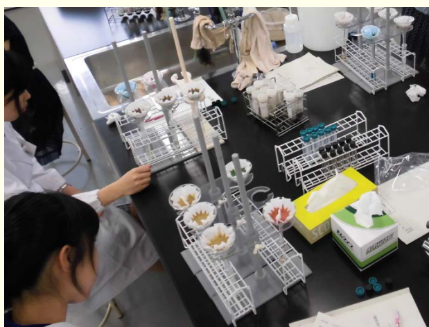
土に未吸着の溶質を含む溶液のろ過
