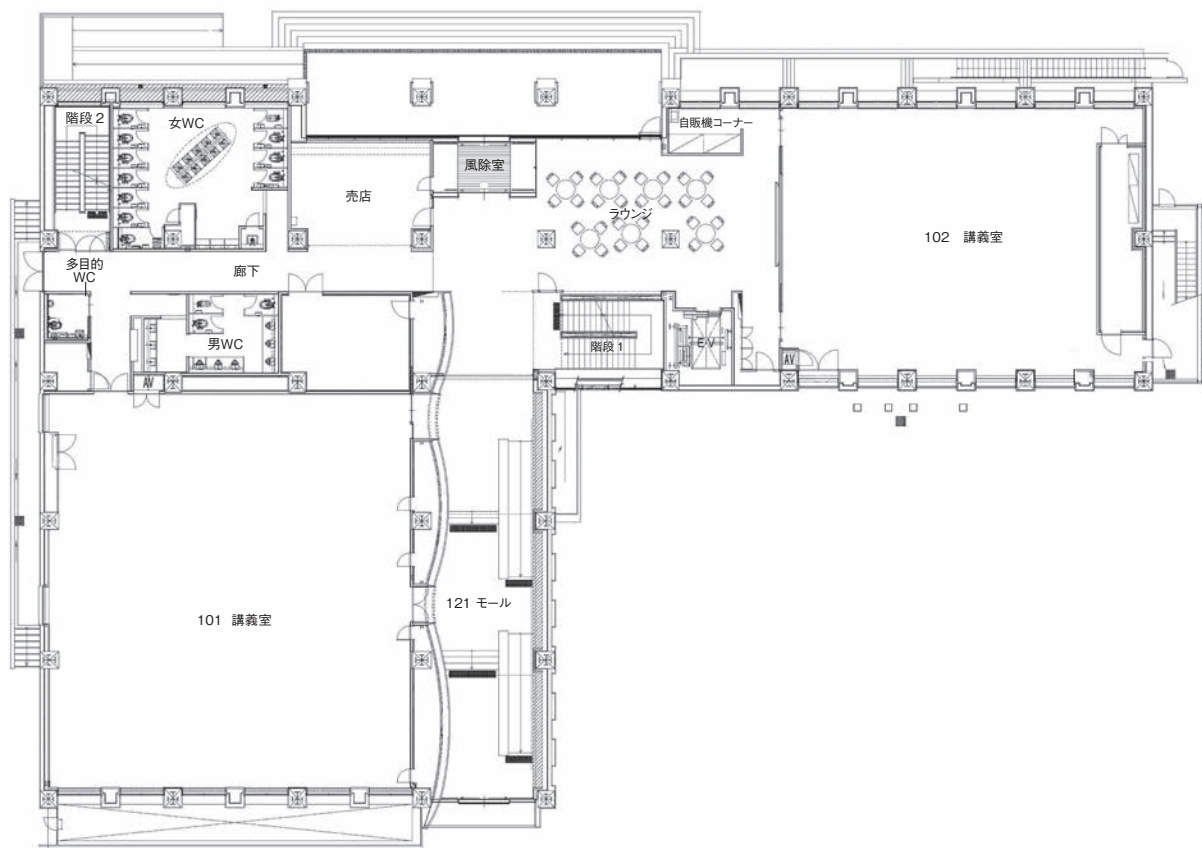
1階
