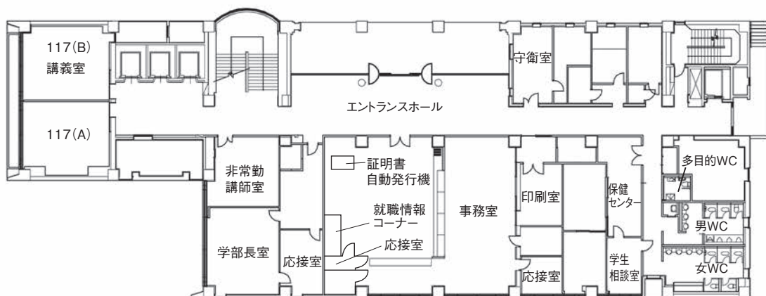
1階
