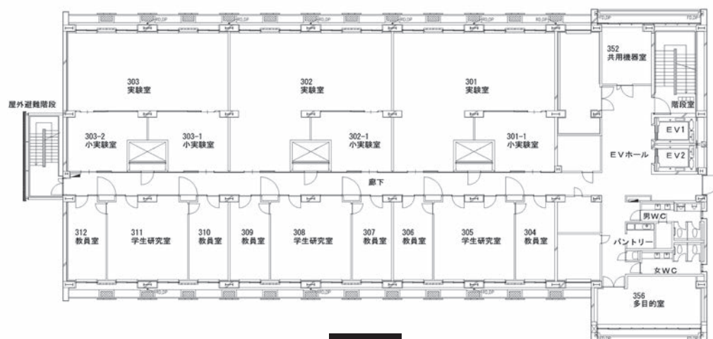
3階
