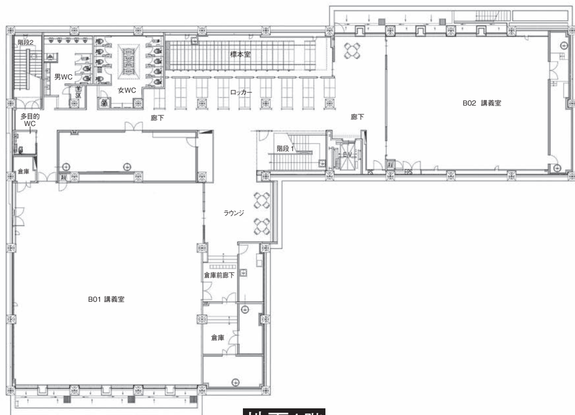
地下1階
