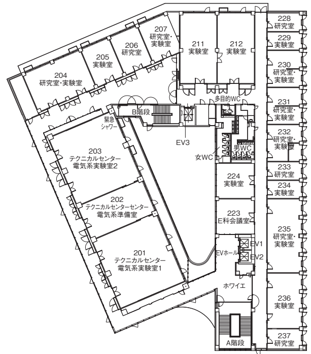
2階
